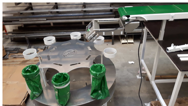
Combinatie met aanvoerband en draaitafel
